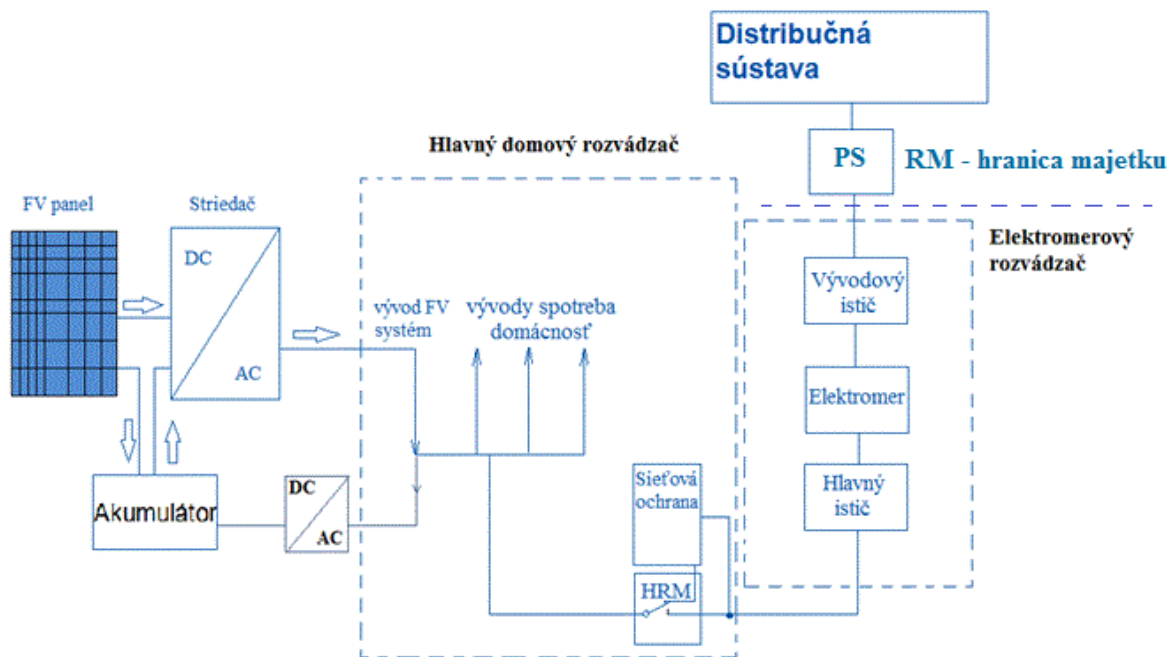
Obrázok 7: Principiálna schéma hybridného systému
