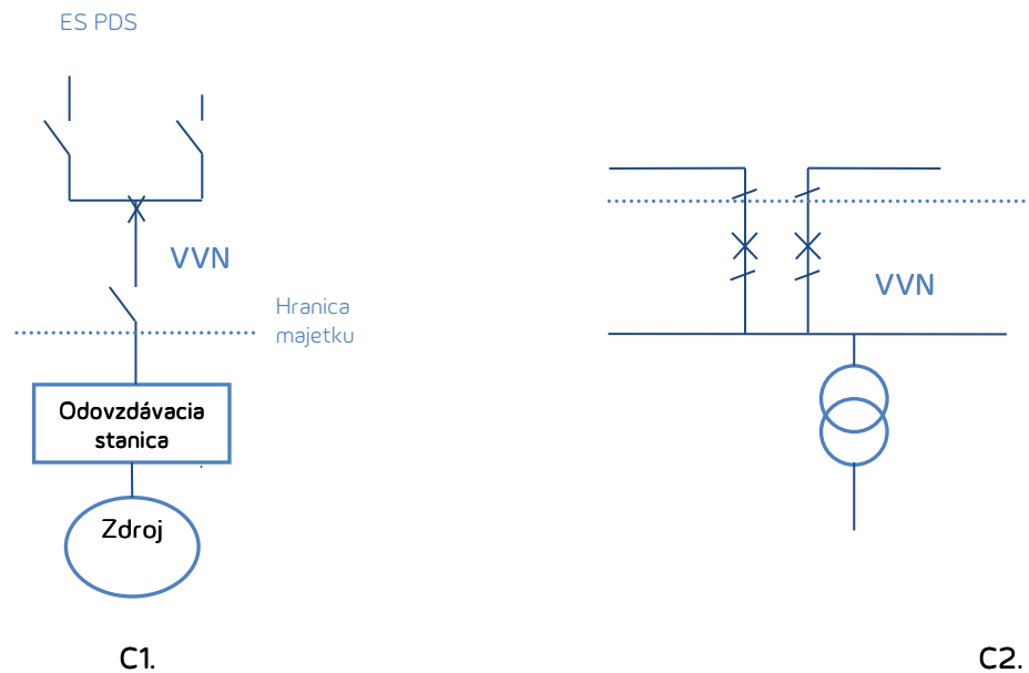
Obrázok 5: Pripojenie zdroja na výrobu elektriny do VVN sústavy
